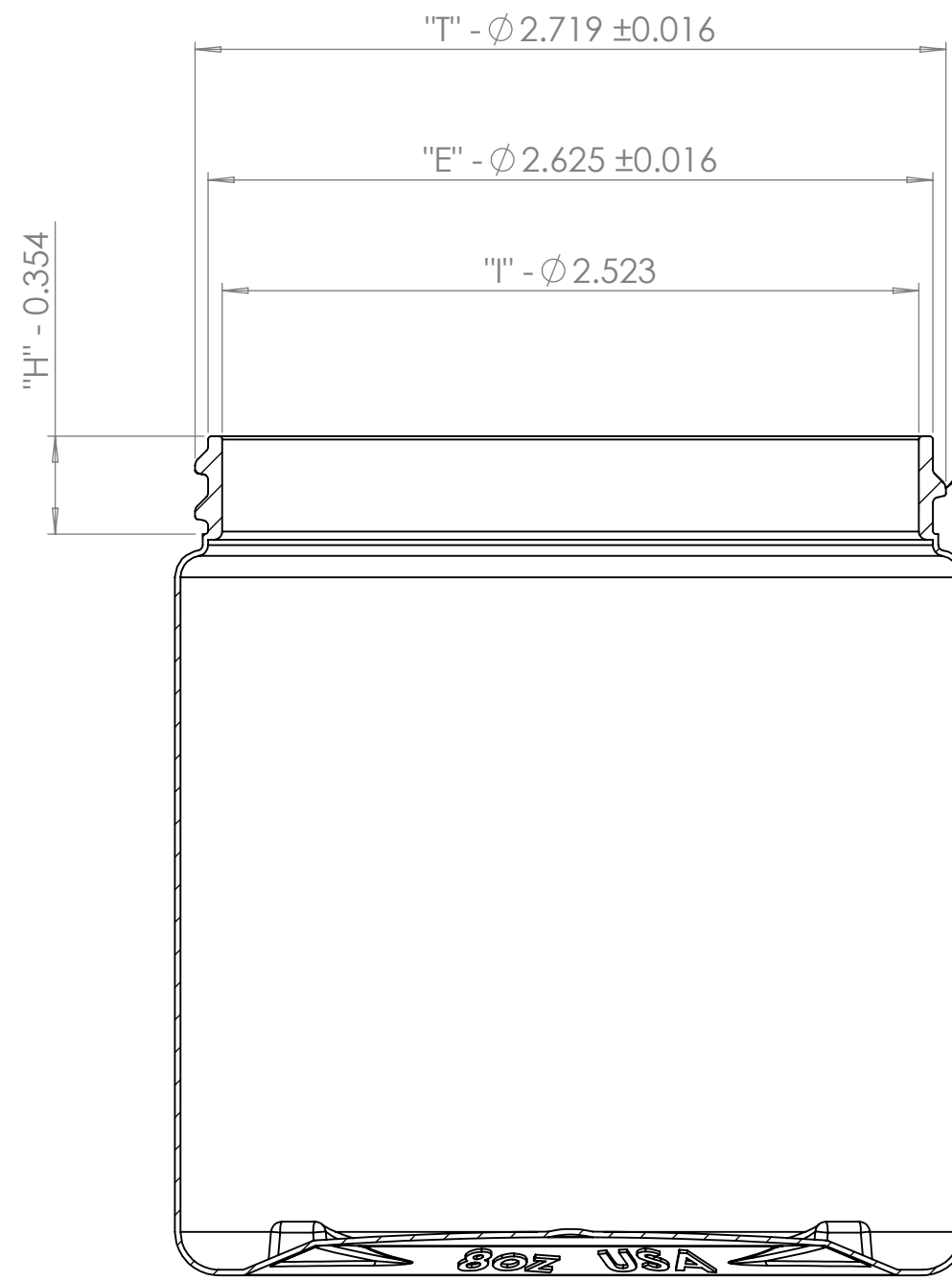
SECTION A-A
